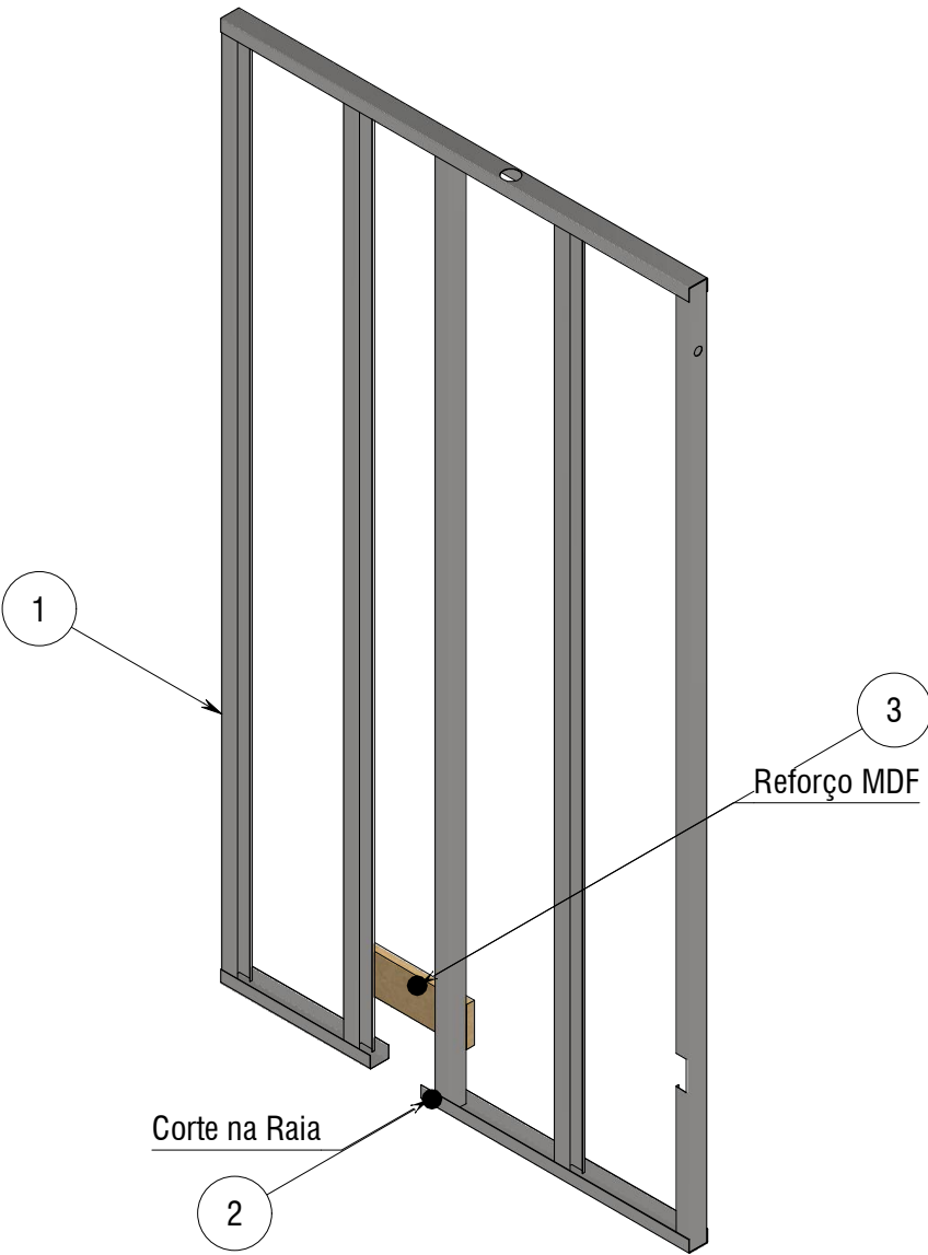
ISOMÉTRICO ( 1 : 15 )
