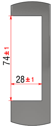
CORTE PARCIAL ( 1 : 2 )
