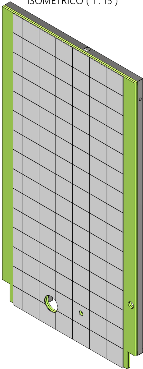
ISOMÉTRICO ( 1 : 15 )
