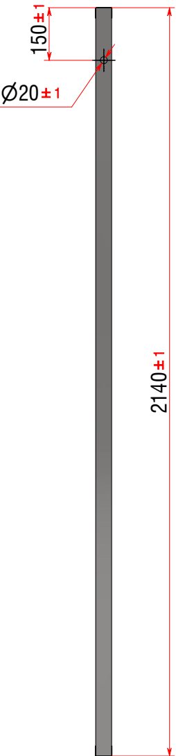
CORTE PARCIAL ( 1 : 2 )
