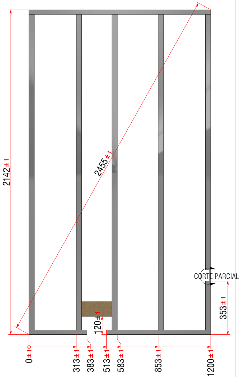
FRENTE ( 1 : 15 )
